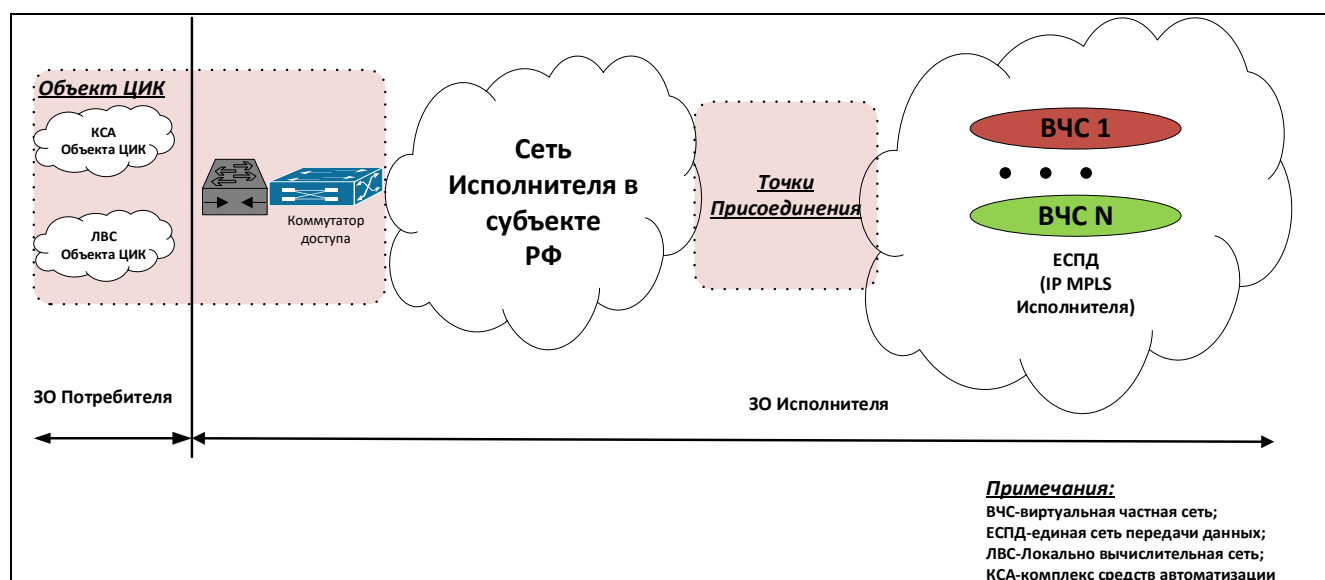
Рис.4.Архитектура Компонента Услуг связи «Передача данных» для Объектов ЦИК.
